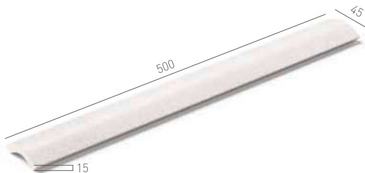
3. Scoth outer corner · Escocia cantonera exterior · MDCA EE00 4.5x4.5
