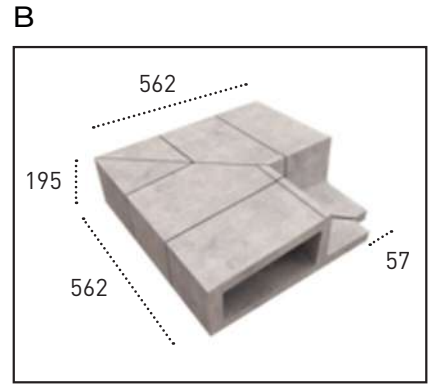
ESQUINA EXTERIOR Ref. SISTEMA BLOCK EE 25
